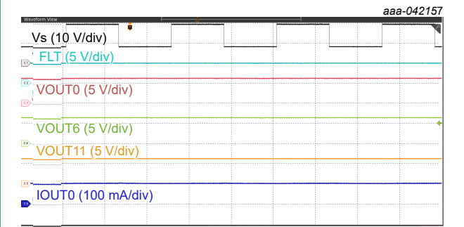
Fig. 19. Vs transient
