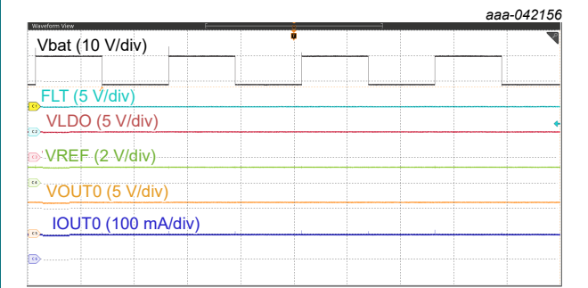
Fig. 18. Vbat transient
