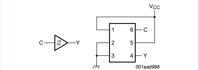
Fig. 7. Buffer
