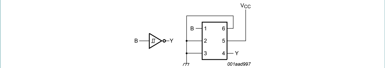
Fig. 8. Inverter
